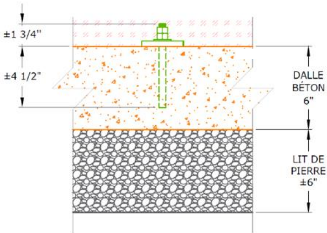
Figure 1 Schéma d'ancrage typique avec tige filetée
